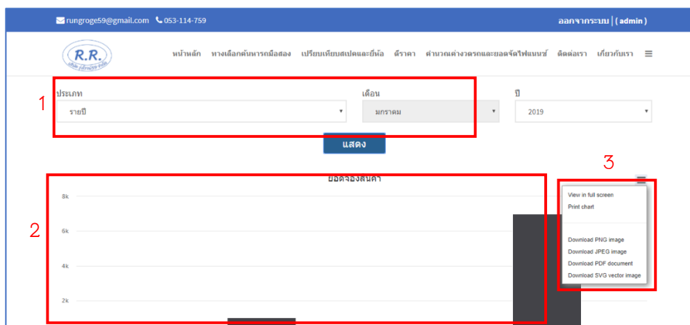
ภาพที่ ก.30 แสดงหน้าจอข้อมูลสถิติการจอง หน้าจอข้อมูลสถิติการจองสามารถเรียกดู ข้อมูลสถิติการจอง ซึ่งประกอบด้วย ส่วนต่าง ๆ ดังนี้ หมายเลข 1 เลือกประเภทข้อมูลสถิติการจองแบบรายเดือนและรายปี หมายเลข 2 ข้อมูลสถิติการจอง หมายเลข 3 ปุ่มสำหรับดาวน์โหลดข้อมูลสถิติการจอง
