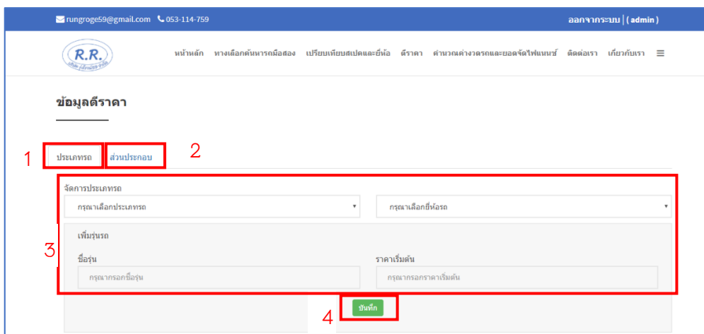
ภาพที่ ก.11 แสดงหน้าจอรายการข้อมูลประเมินราคา หน้าจอข้อมูลประเมินราคาสามารถแก้ไข ข้อมูลราคาของรถได้ ซึ่ง ประกอบด้วยส่วนต่าง ๆ ดังนี้
